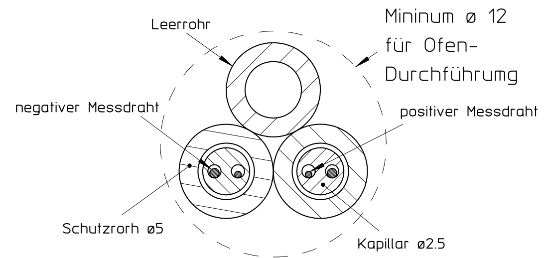
Schnitt A - A 5:1
