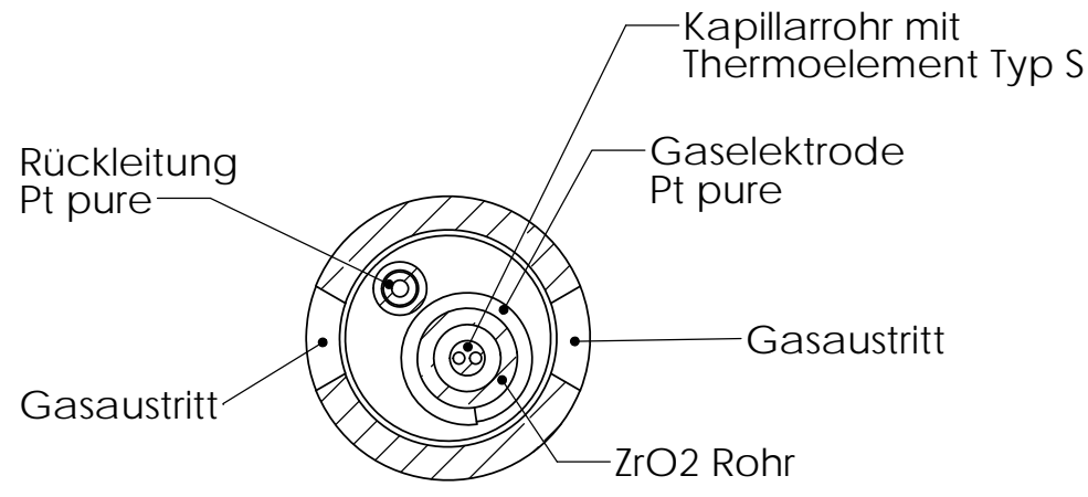
SCHNITT E-E MAßSTAB 2 : 1
